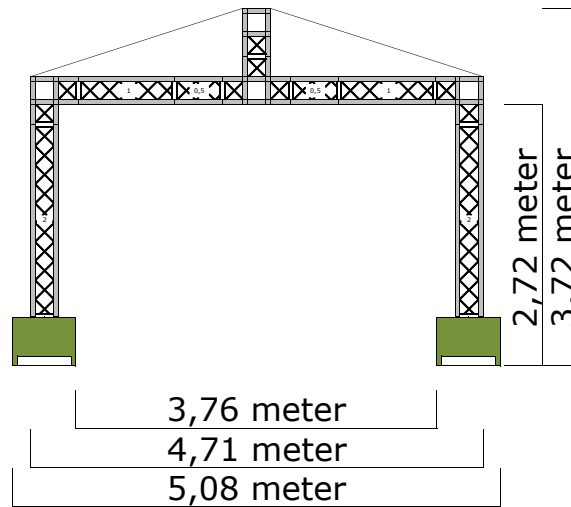
Zij aanzicht
