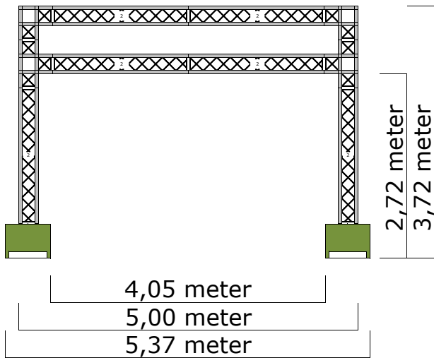
Vooraanzicht
