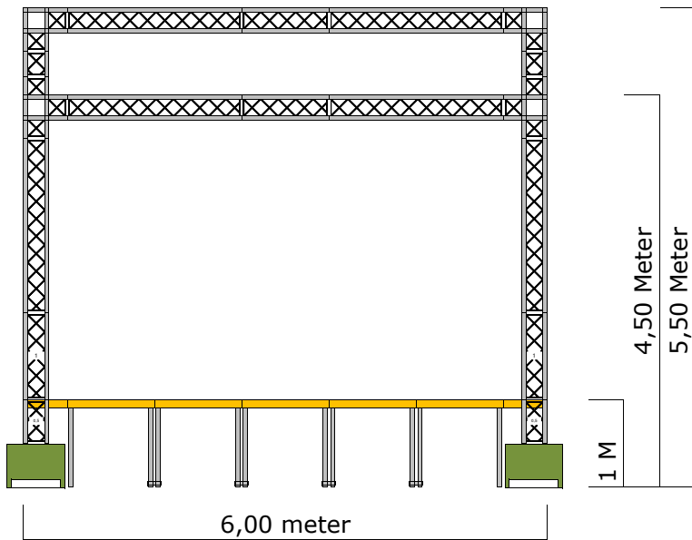
Voor aanzicht
