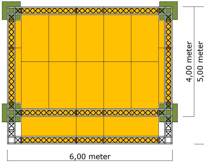
Boven aanzicht
