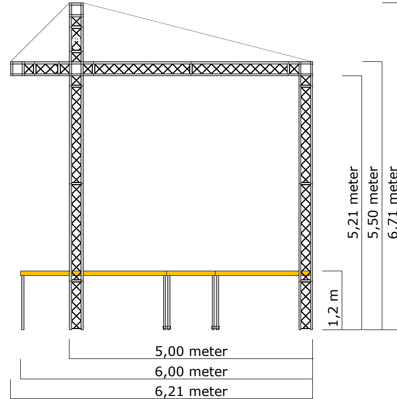
Zij aanzicht
