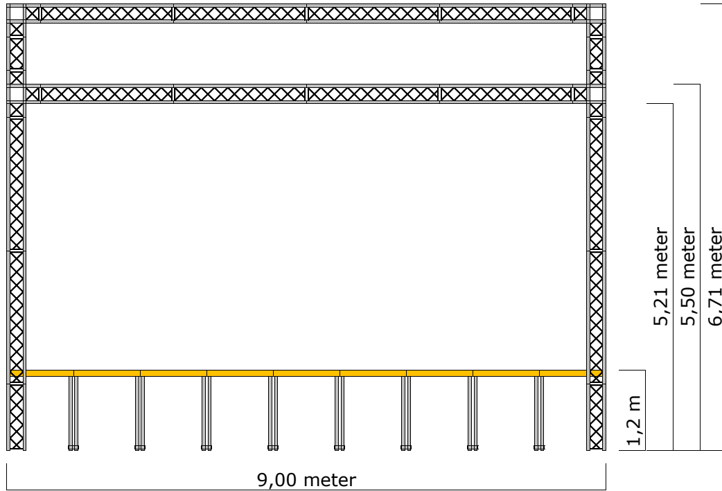
Voor aanzicht
